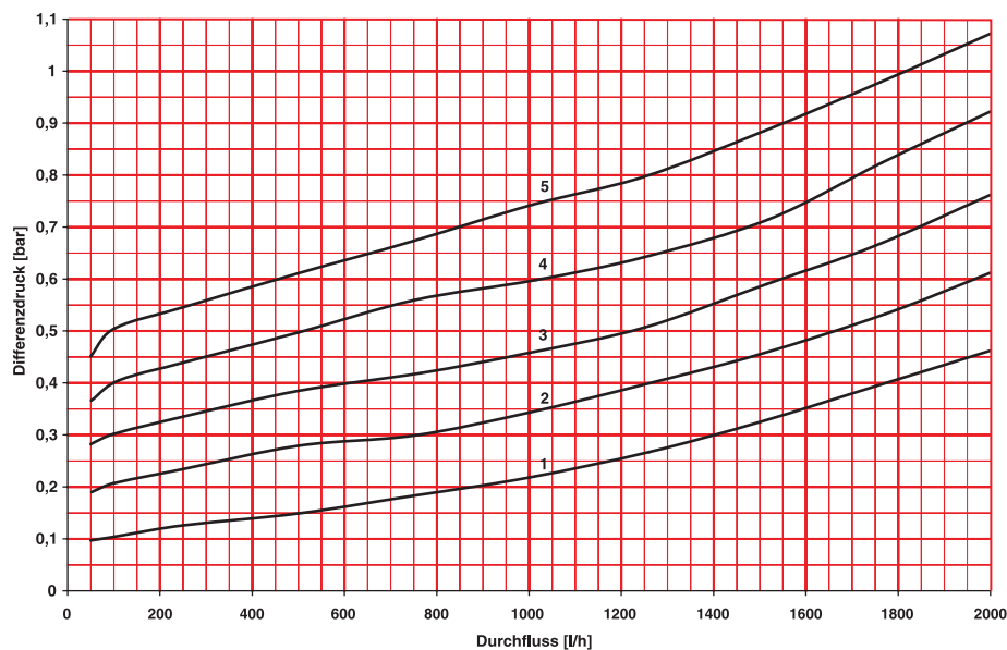
4004 dp / Q-Diagramm
