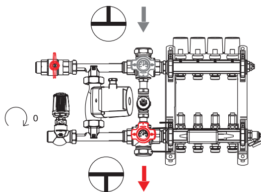
Heizkreisspülung
